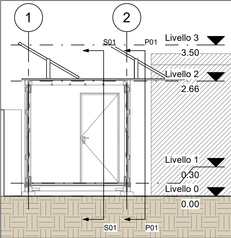
P02 Scala 1 : 50
