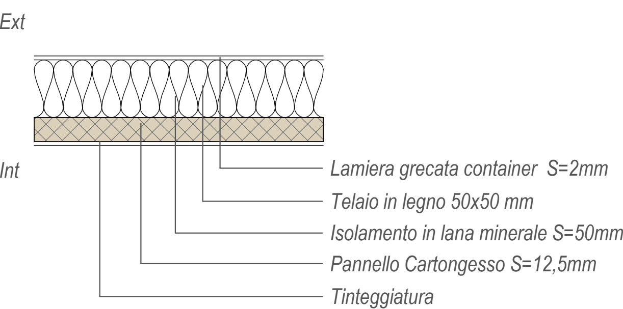
DT03 - Controsoffitto interno
