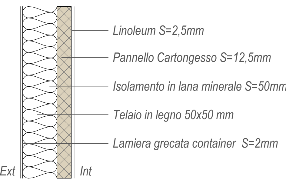
DT01 - Parete perimetrale interna
