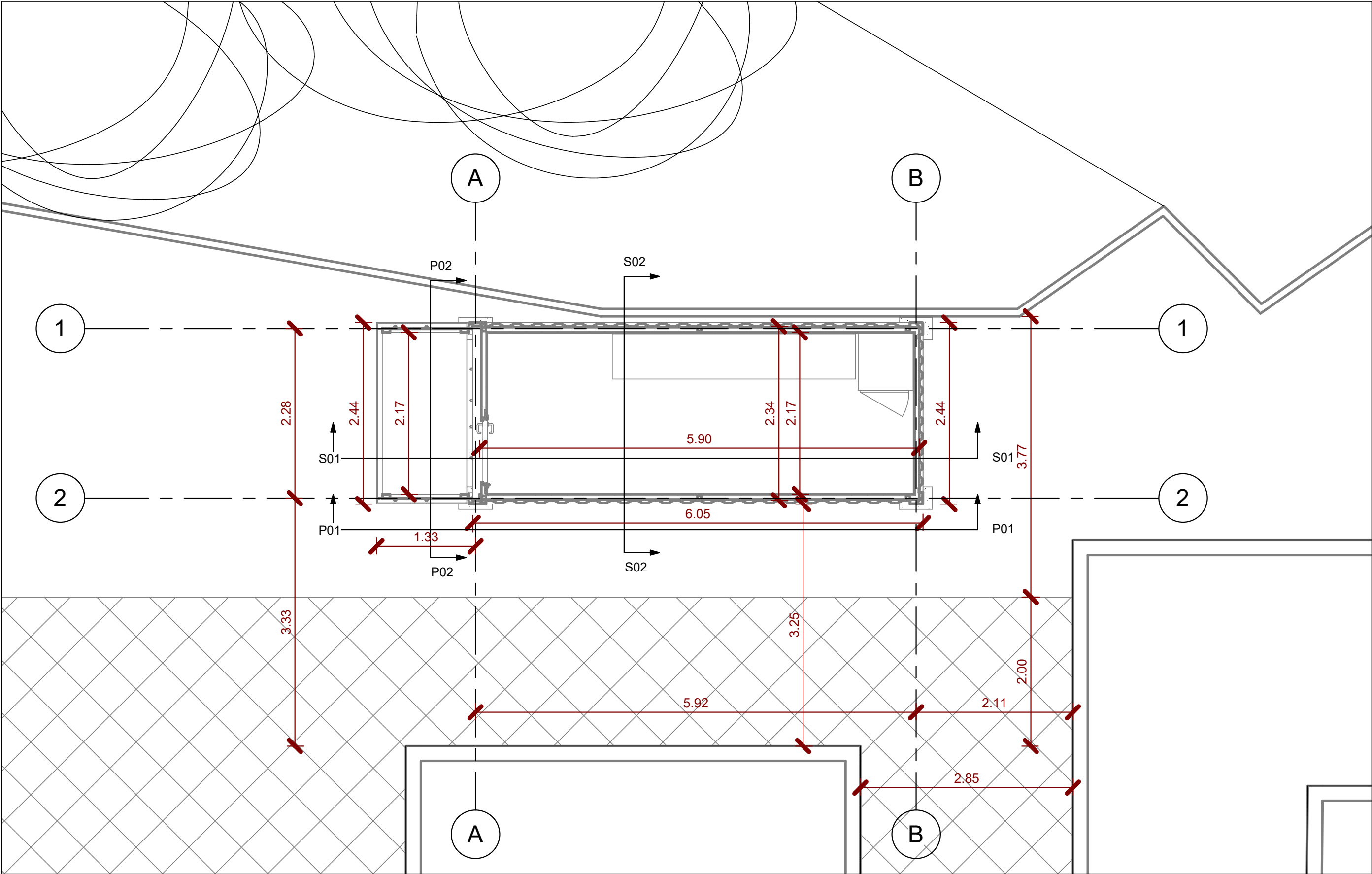
Pianta livello 1 Scala 1 : 50
