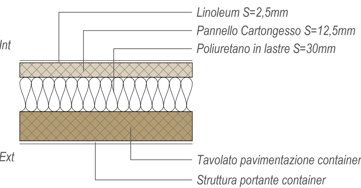
DT04 - Pavimentazione interna
