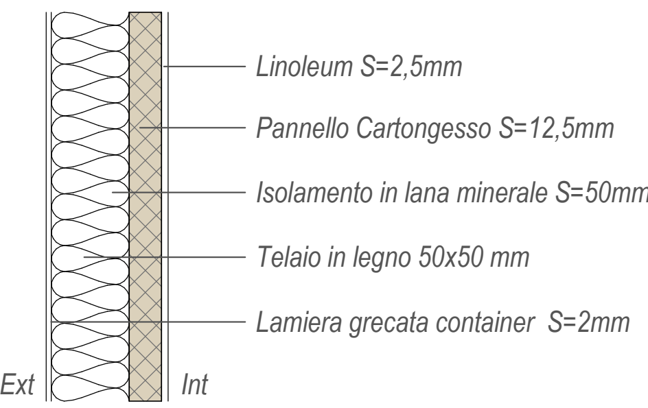
DT02 - Parete interna
