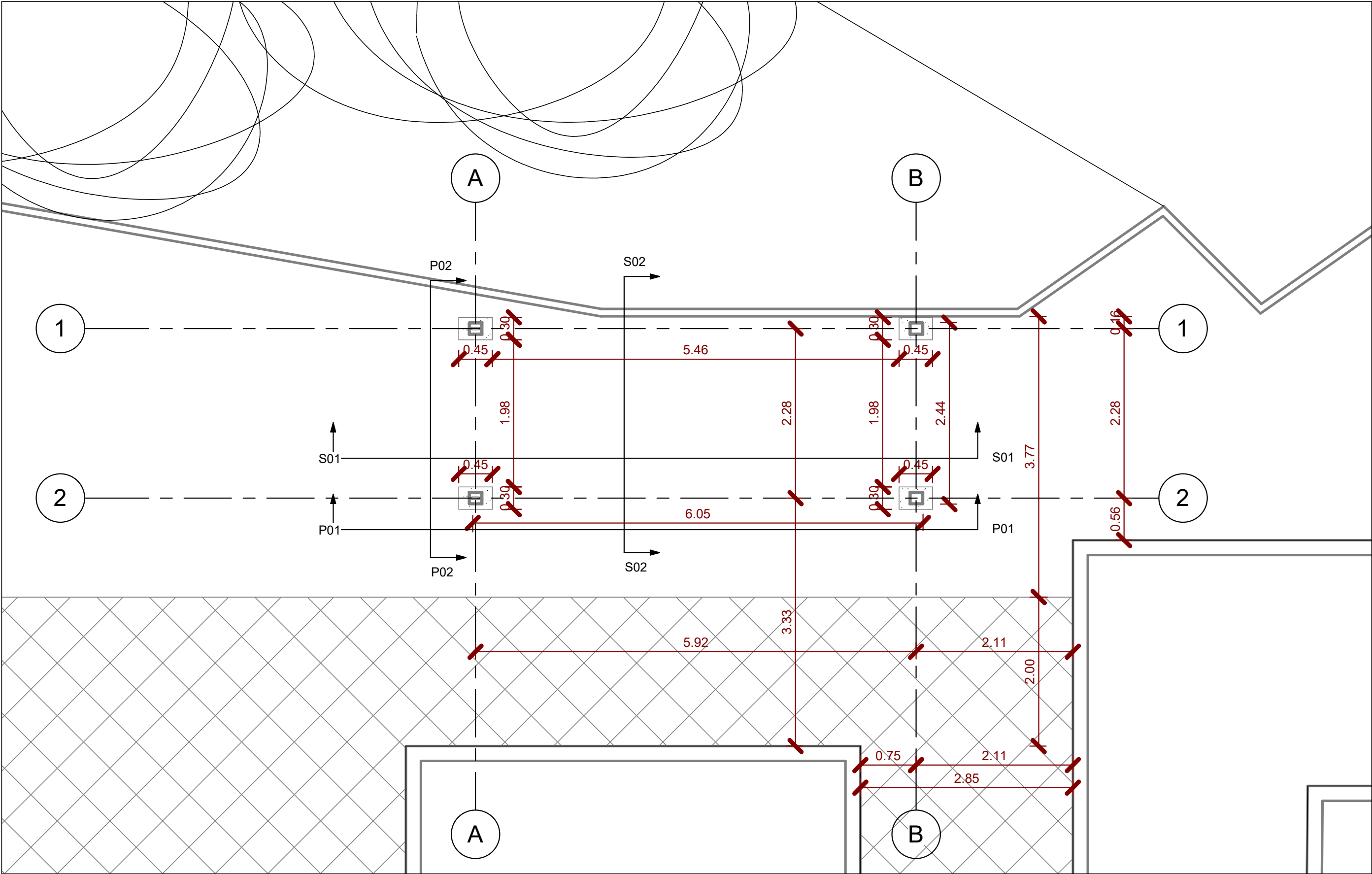
Pianta livello 0 Scala 1 : 50
