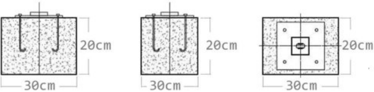
DT05 - Baggioli di fondazione
