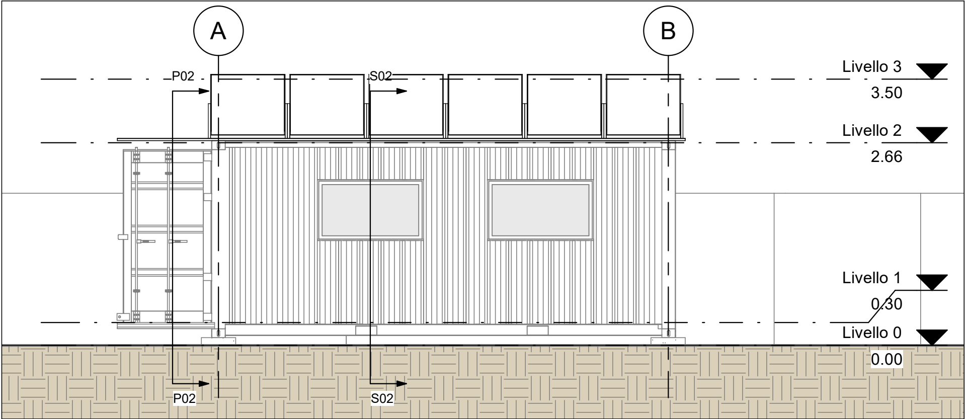
P01 Scala 1 : 50
