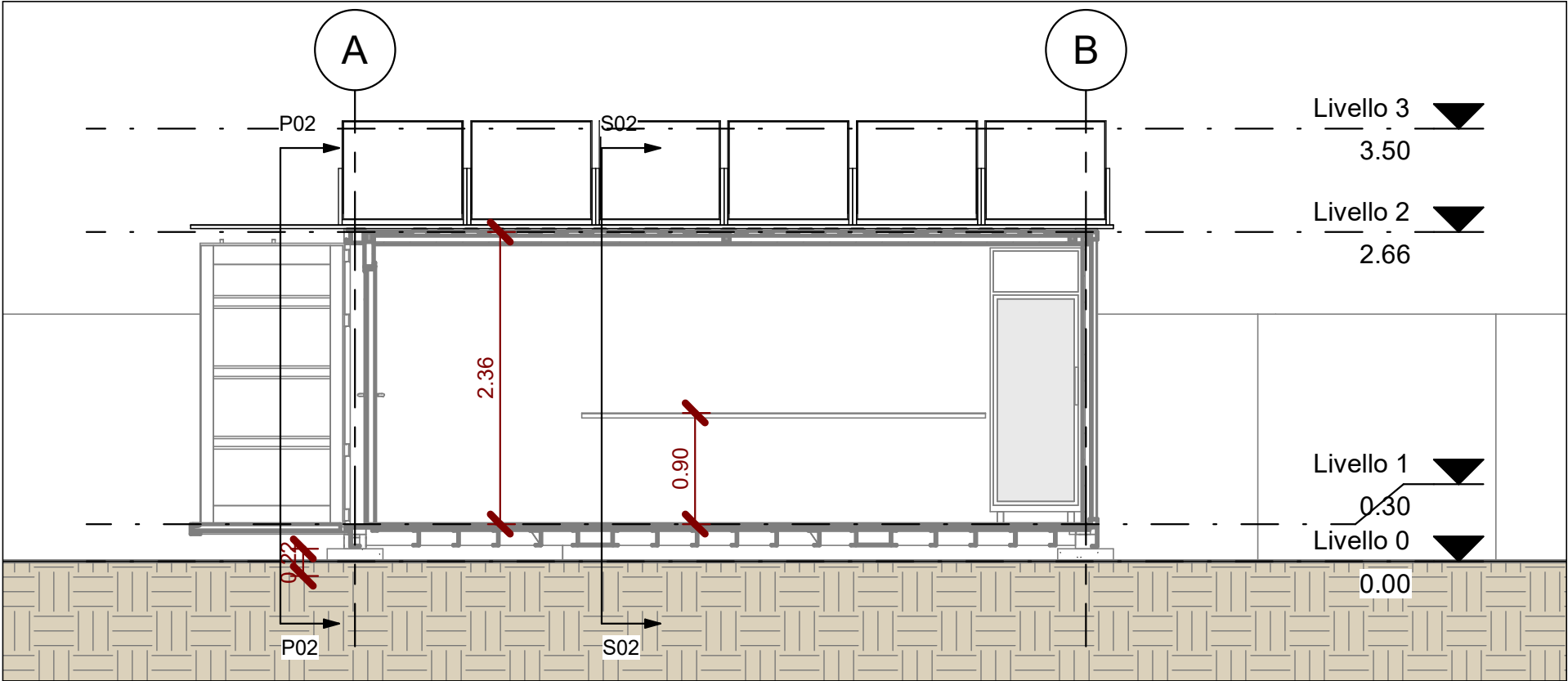
S01 Scala 1 : 50
