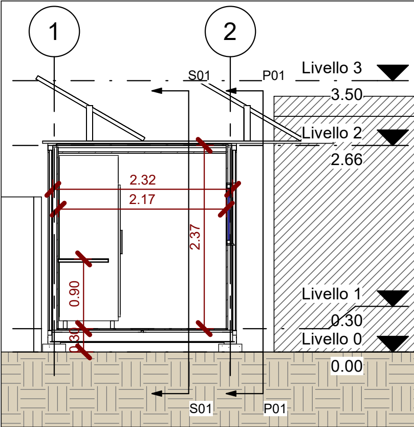
S02 Scala 1 : 50
