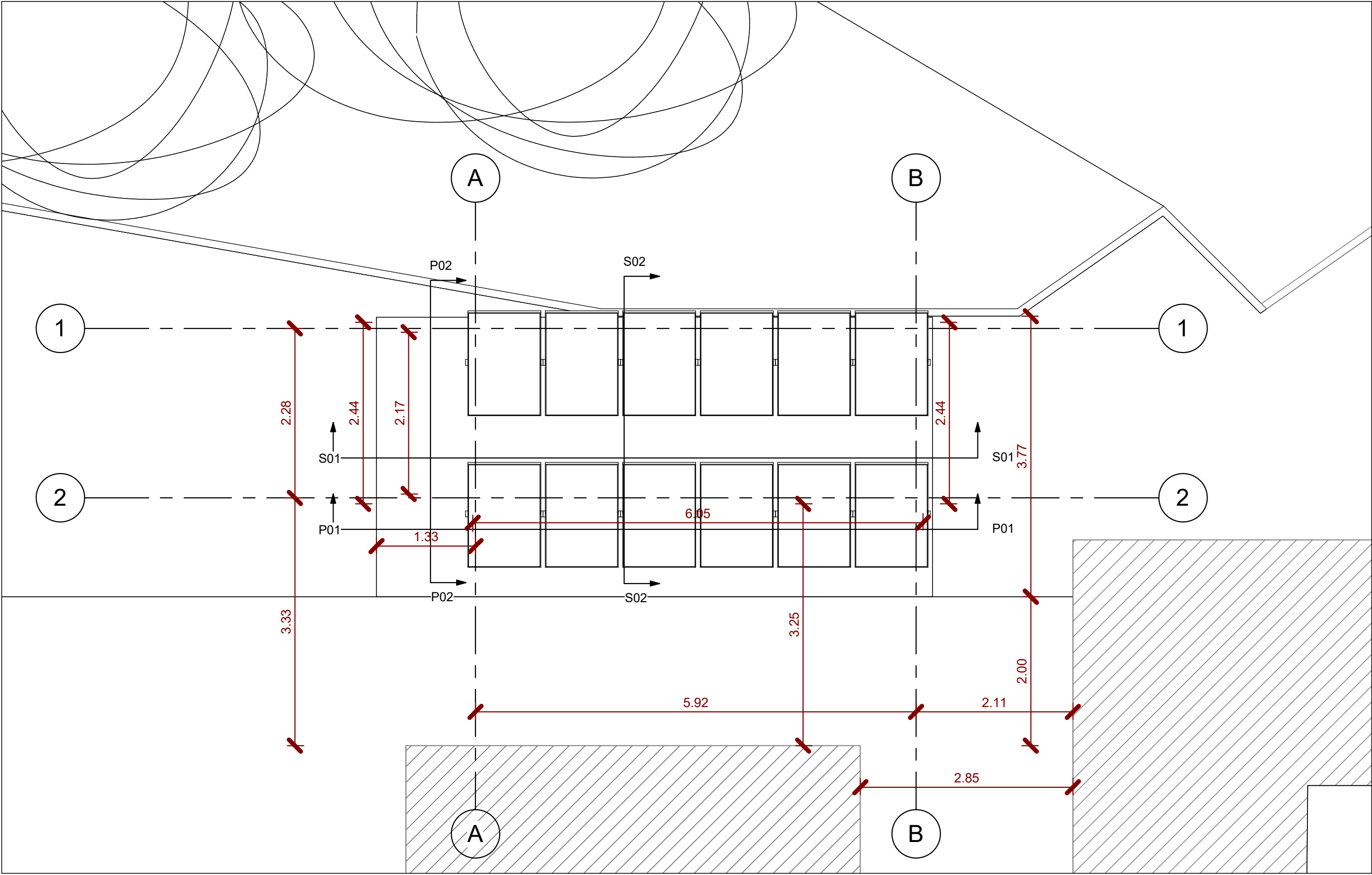
Pianta livello Copertura Scala 1 : 50
