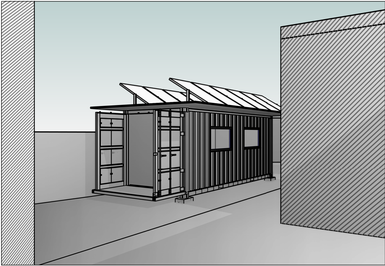
Vista 3D - A_posa pannelli Scala
